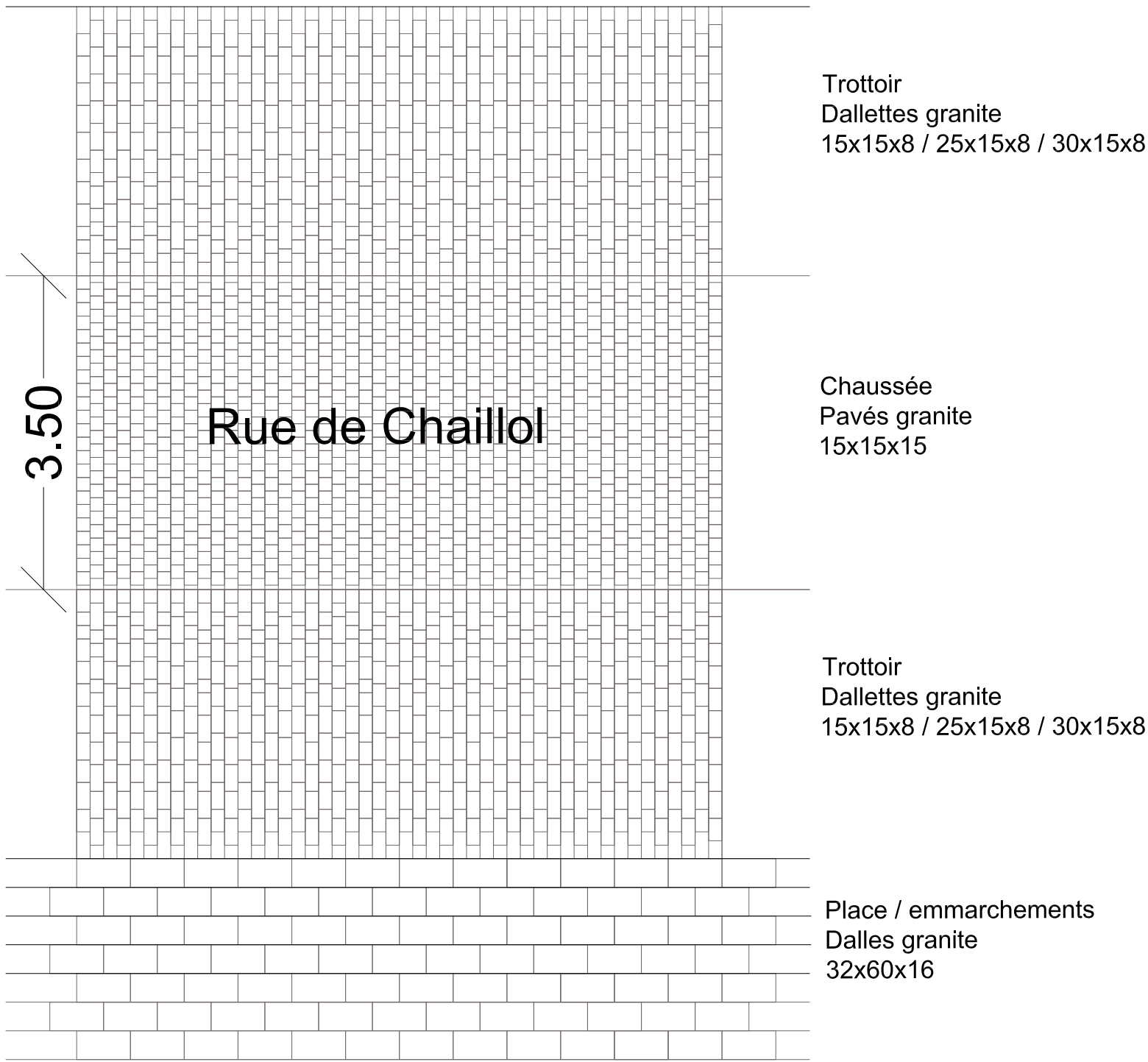
Plan de détails du calepin
