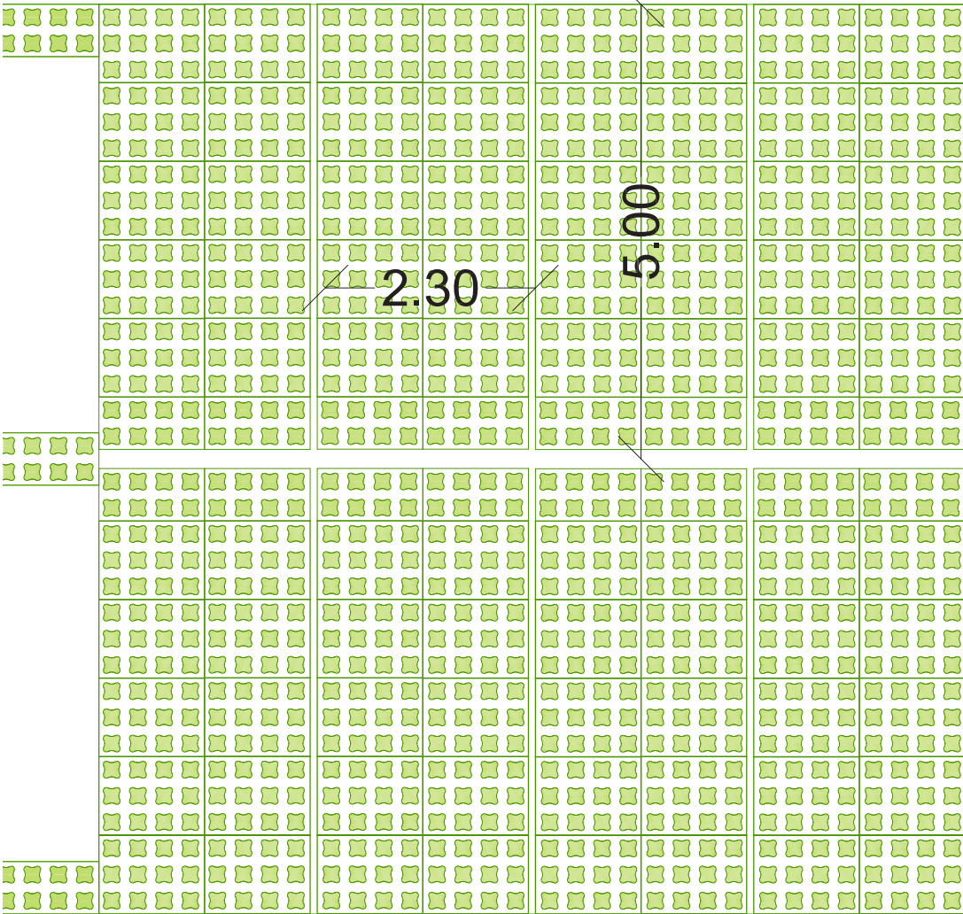
Plan de calepinage
